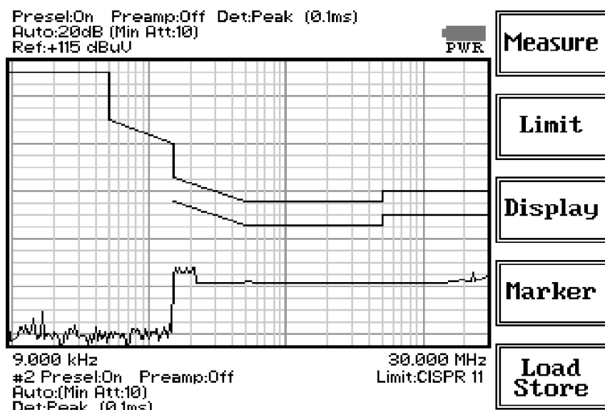
Fig. 4-1 Sweep
