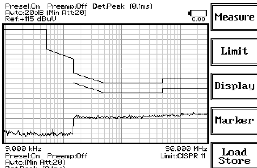
Fig. 15-2 Sweep
