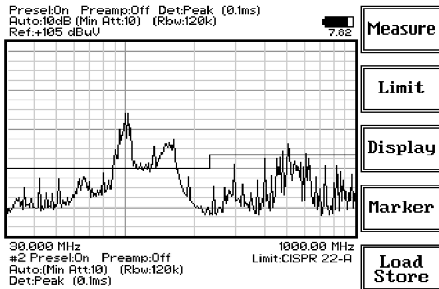
Fig. 11-18 Sweep
