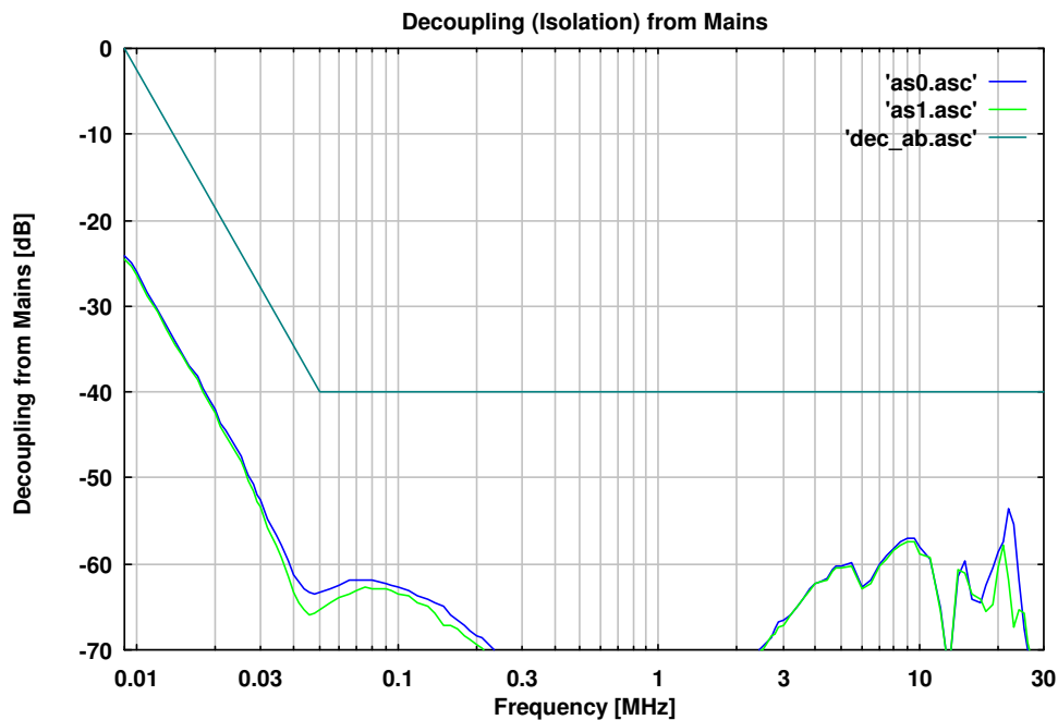
Abb. 6 Entkopplung vom Speisetz (Prüflingsklemmen) Fig. 6 Decoupling from power supply (EuT terminals)
