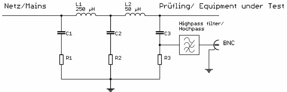
Abb. 1 NSLK 8127 Netznachbildung mit Option PLC, nur ein Pfad dargestellt Fig.1 NSLK 8127 Artificial Mains Network with option PLC, only one path shown
