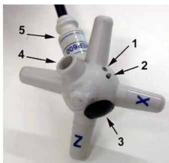
Рис.1-7 Пластиковый корпус
