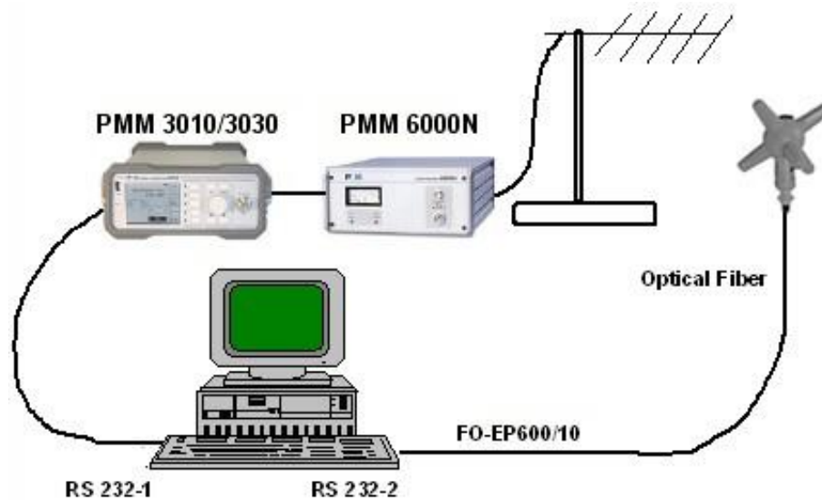
Рис. 3-1 PMM EP60x открытая испытательная площадка
