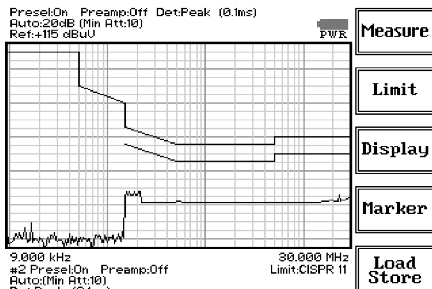
Fig. 4-1 Sweep
