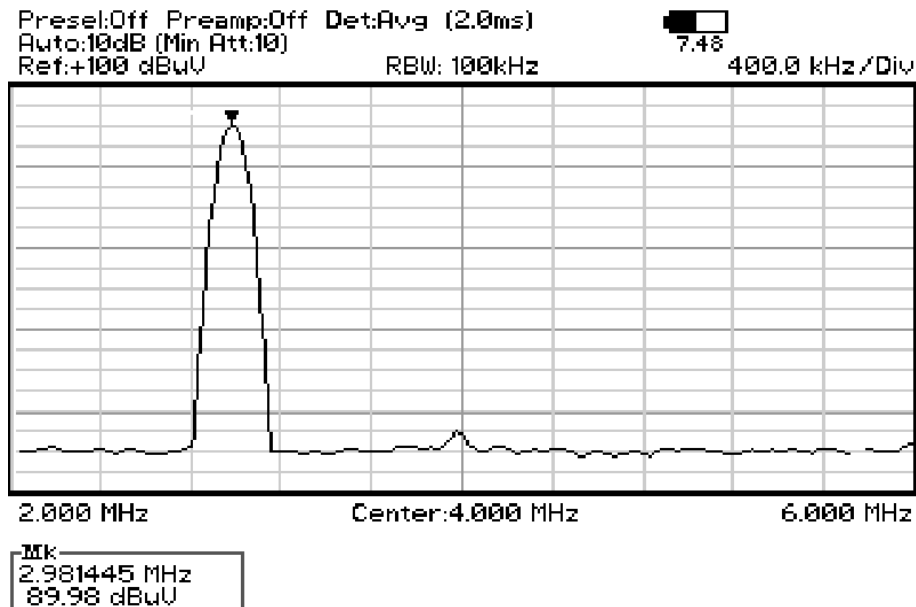
Fig. 15-3 Spectrum
